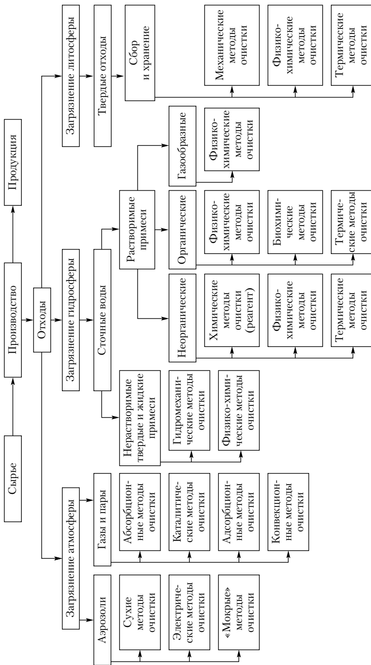
Рис. 1.1. Схема обезвреживания и переработки промышленных отходов
